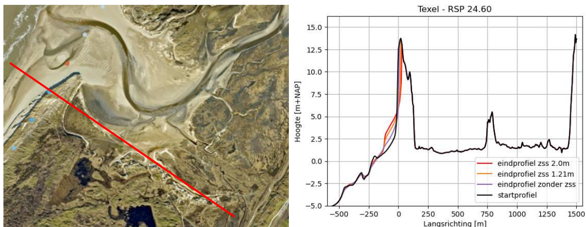
Figuur 19 Afslagprofielen voor de Jarkusraai bij RSP 24.60 op het eiland Texel. Links is de locatie weergegeven in rood op een satellietbeeld uit 2023. Rechts het startprofiel in zwart en een afslagprofiel voor het huidige zichtjaar zonder zeespiegelstijging (paars), een afslagprofiel met 1,21m zeespiegelstijging in 2100 (oranje) en een afslagprofiel met 2,0m zeespiegelstijging in 2100 (rood). Met de iconen zijn de objecten aangegeven.
