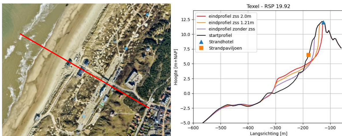
Figuur 18 Afslagprofielen voor de Jarkusraai bij RSP 19.92 op het eiland Texel. Links is de locatie weergegeven in rood op een satellietbeeld uit 2023. Rechts het startprofiel in zwart en een afslagprofiel voor het huidige zichtjaar zonder zeespiegelstijging (paars), een afslagprofiel met 1,21m zeespiegelstijging in 2100 (oranje) en een afslagprofiel met 2,0m zeespiegelstijging in 2100 (rood). Met de iconen zijn de objecten aangegeven.
