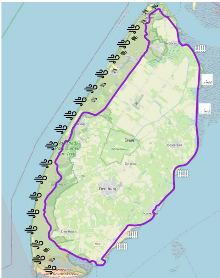
Figuur 27 Locaties waar doorstuiving (windvaantjes), waar meegroei van voorlanden (لاند) en waar luwte (hekjes) t.b.v. meegroei gestimuleerd kan worden binnen ambitieniveau 3. In paars de primaire kering.
