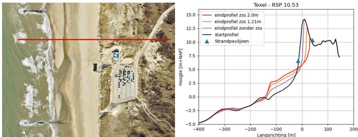
Figuur 17 Afslagprofielen voor de Jarkusraai bij RSP 10.53 op het eiland Texel. Links is de locatie weergegeven in rood op een satellietbeeld uit 2023. Rechts het startprofiel in zwart en een afslagprofiel voor het huidige zichtjaar zonder zeespiegelstijging (paars), een afslagprofiel met 1,21m zeespiegelstijging in 2100 (oranje) en een afslagprofiel met 2,0m zeespiegelstijging in 2100 (rood). Met de iconen zijn de objecten aangegeven.
