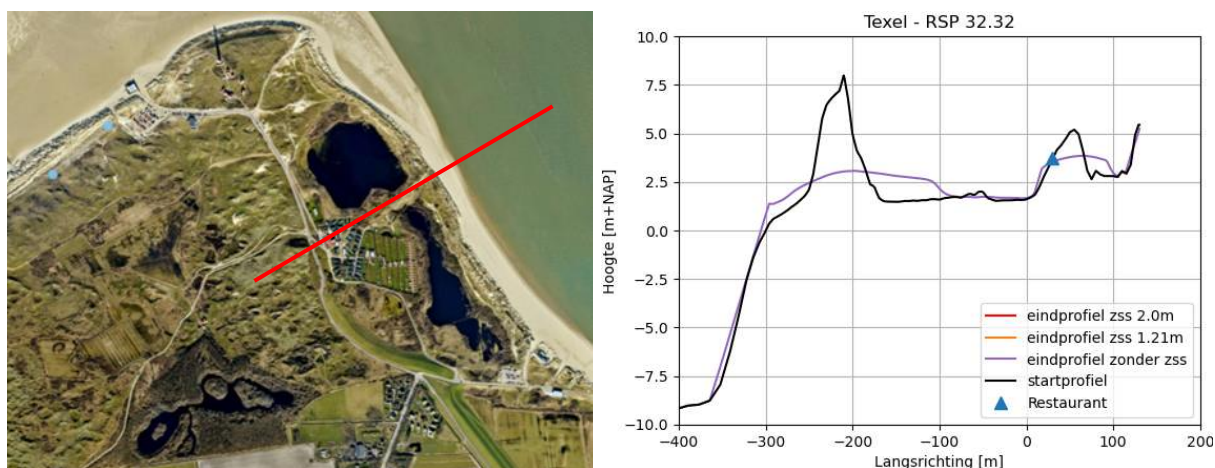
Figuur 20 Afslagprofielen voor de Jarkusraai bij RSP 32.32 op het eiland Texel. Links is de locatie weergegeven in rood op een satellietbeeld uit 2023. Rechts het startprofiel in zwart en een afslagprofiel voor het huidige zichtjaar zonder zeespiegelstijging (paars), een afslagprofiel met 1,21m zeespiegelstijging in 2100 (oranje) en een afslagprofiel met 2,0m zeespiegelstijging in 2100 (rood). Met de iconen zijn de objecten aangegeven.
