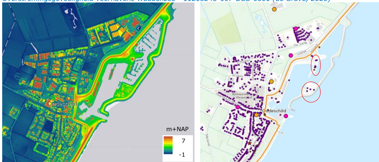
Figuur 23 Kustprofiel Oudeschild Texel – Interessesgebied overstromingsgevoeligheid
