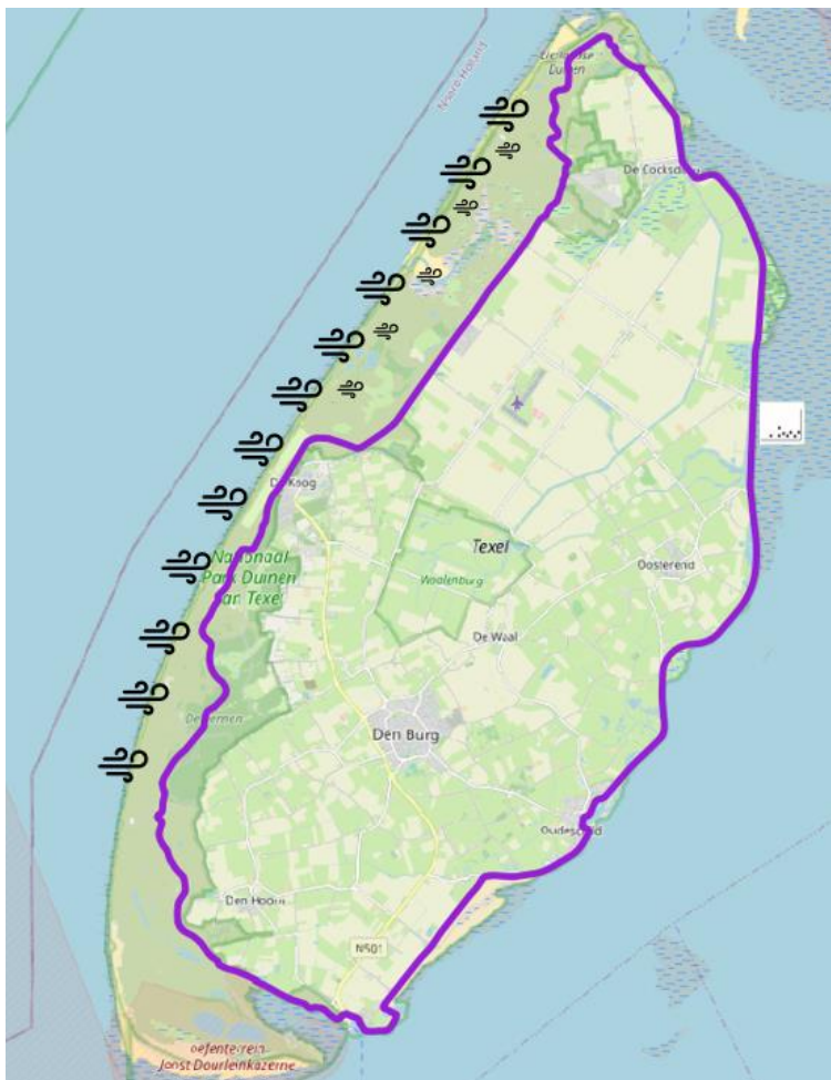
Figuur 26 Locaties waar doorstuiving (windvaantjes) en waar meegroeien van voorlanden (البحر) gestimuleerd kan worden binnen ambitieniveau 2. In paars de primaire kering.
